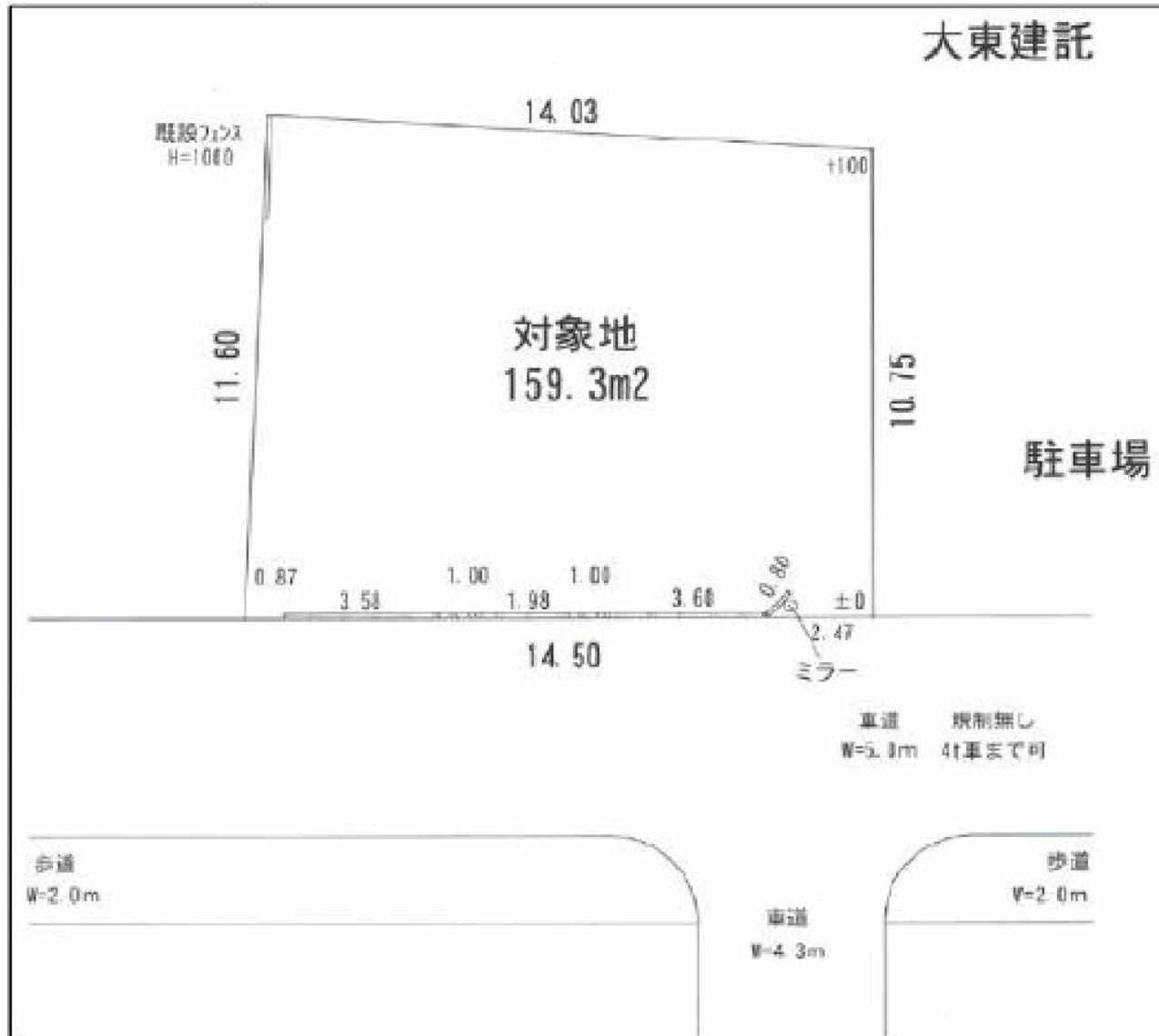
現場平面図
